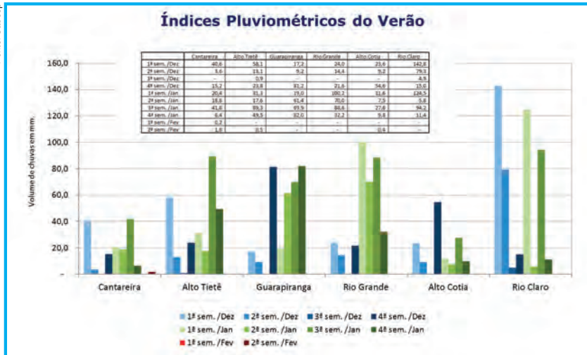
Varição dos índices pluviométricos de dezembro a fevereiro, nos diferentes sistemas de captação de água do Estado de São Paulo
