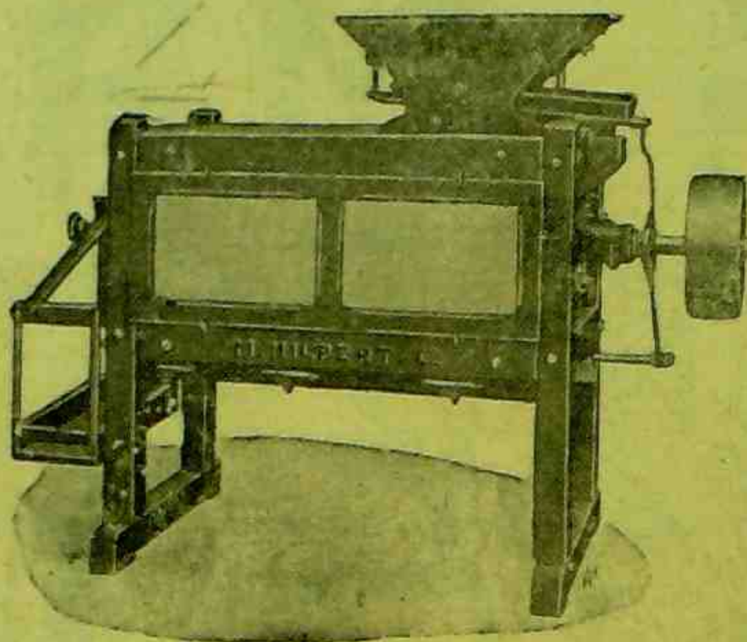
Moinho combinado com Classificador e Separador Especial
