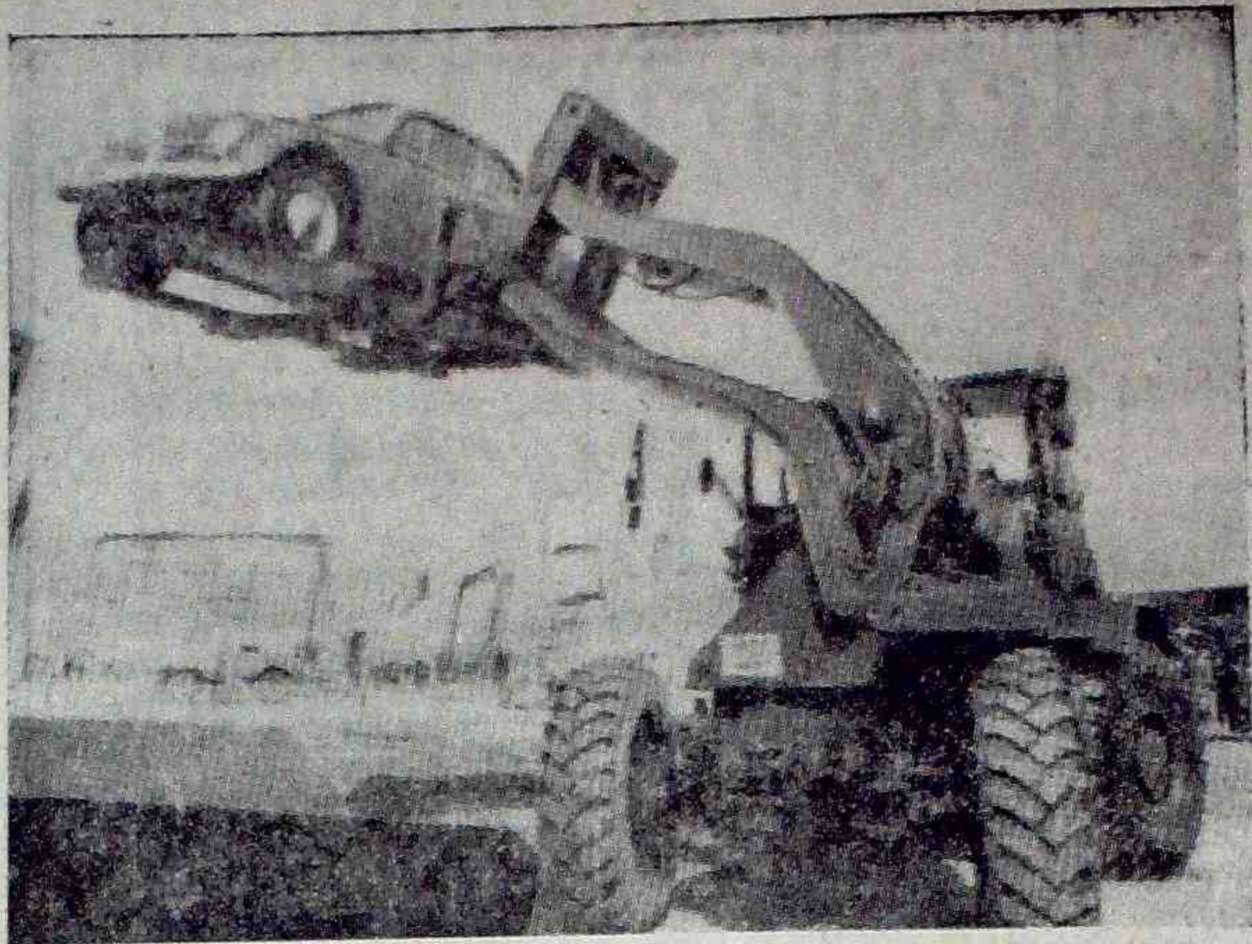
Na exposição da BAUMA, em Munique, foram exibidas experiências com um elevador de carga que pode suspender lateralmente um automóvel para o ar.
